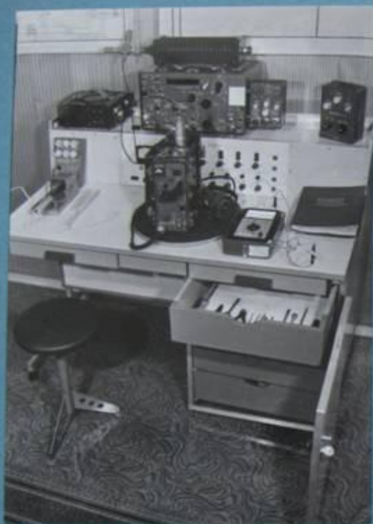
Общий вид поста для проведения ремонта и регламентных работ
